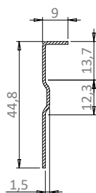
A-A METSZET
