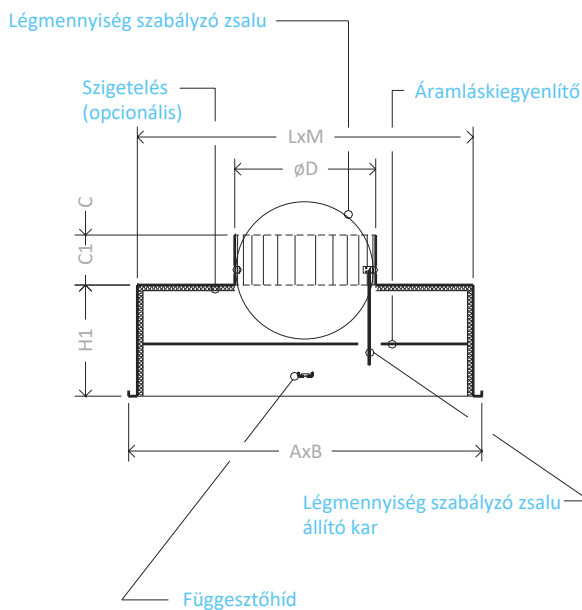
Felső csatlakozással (P2)
