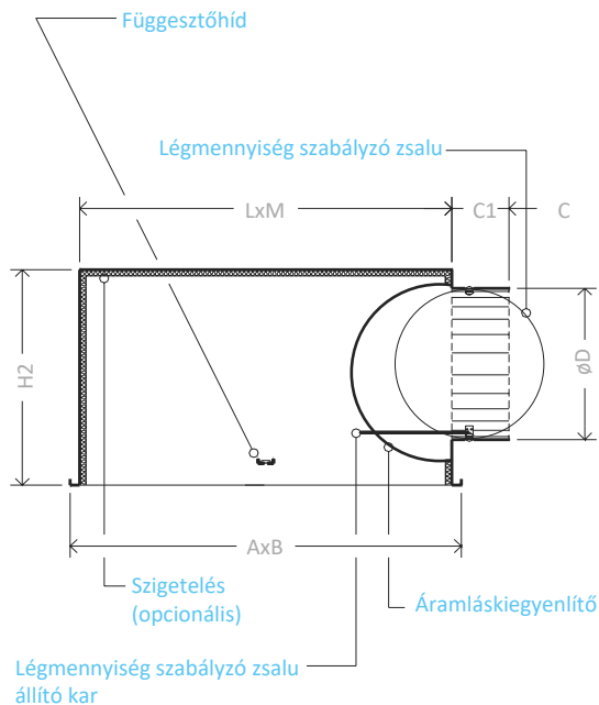
Oldalsó csatlakozással (P1)
