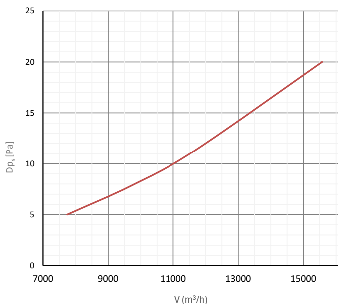
Statikus nyomásvesztés
