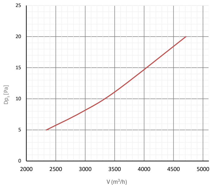
Statikus nyomásvesztés
