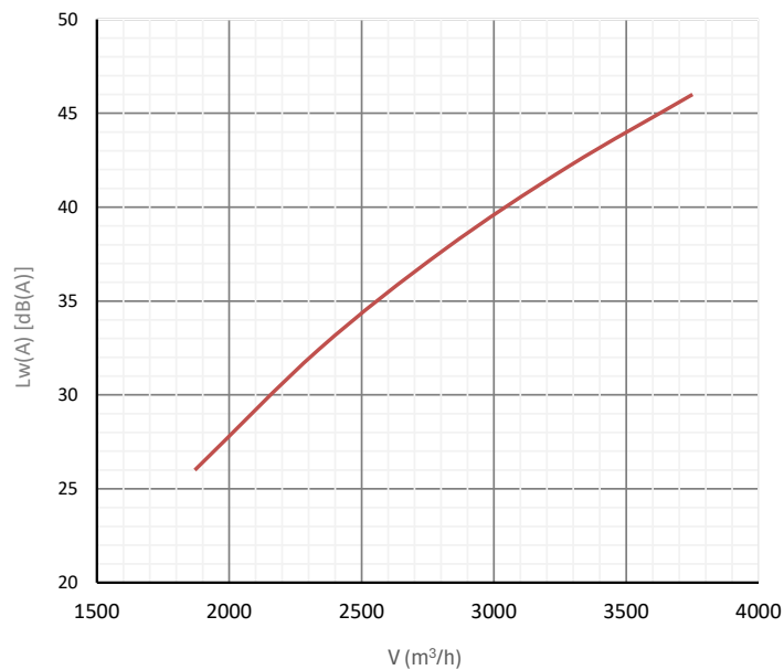
Hangteljesítményszint
