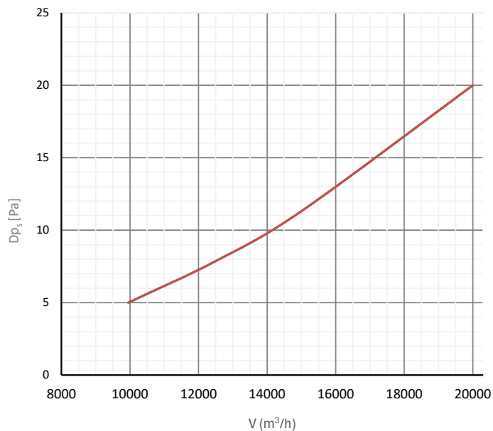
Statikus nyomásvesztés
