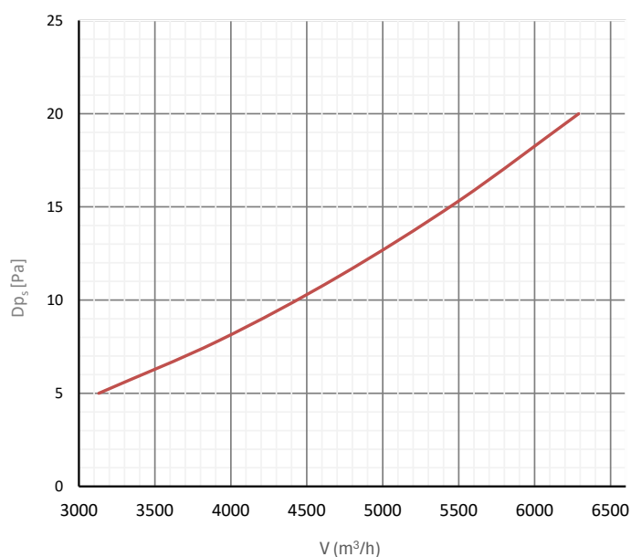
Statikus nyomásvesztés
