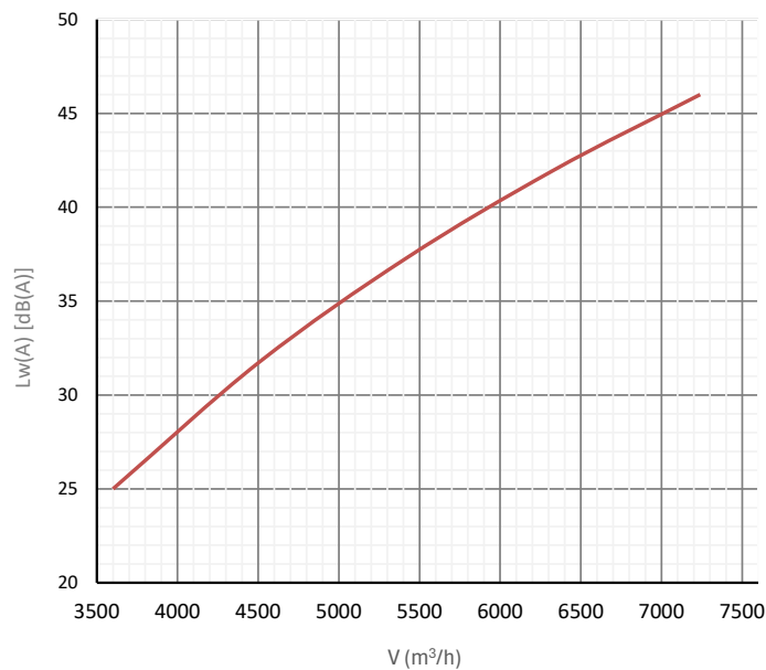
Hangteljesítményszint
