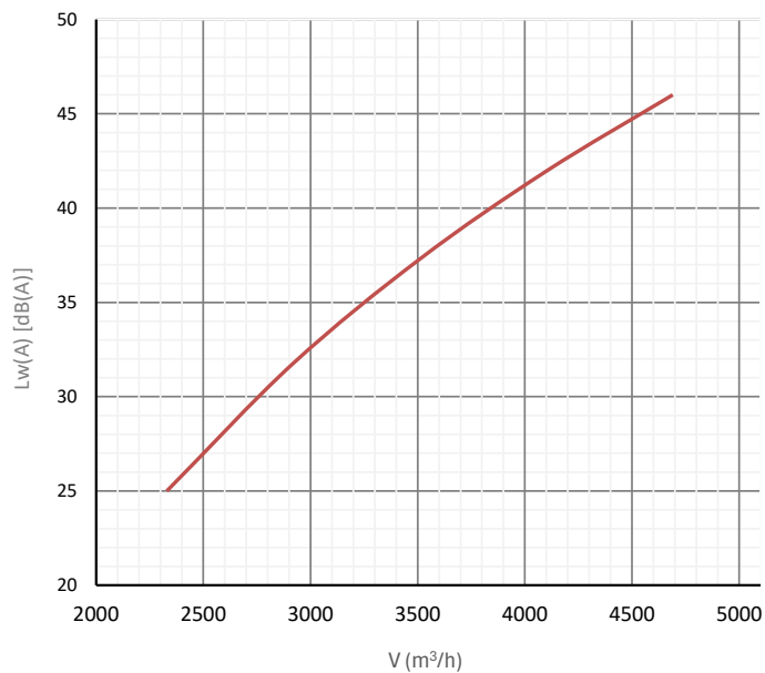
Hangteljesítményszint
