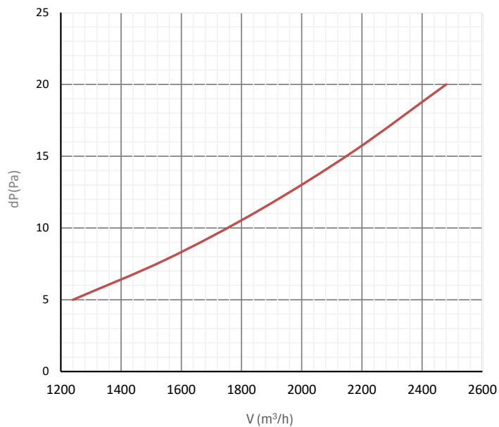
Statikus nyomásvesztés
