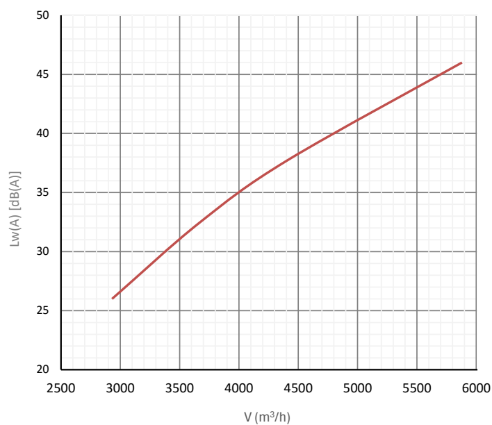
Hangteljesítményszint
