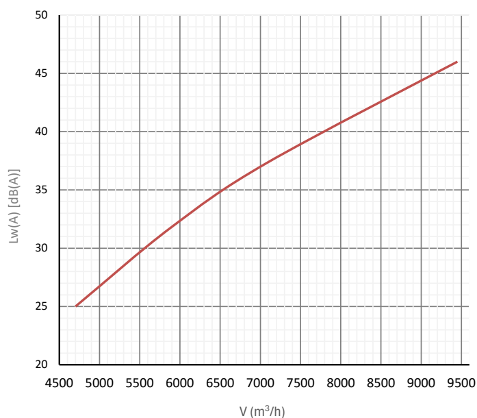
Hangteljesítményszint
