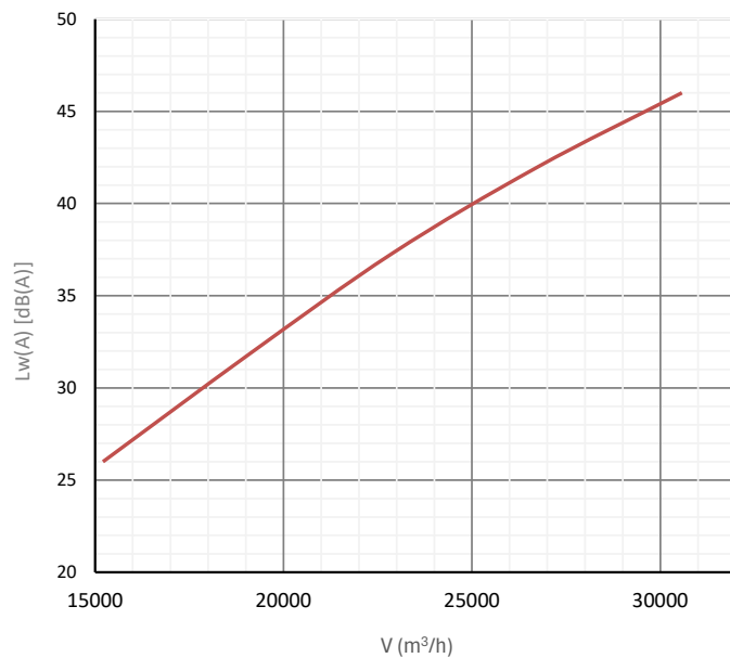
Hangteljesítményszint
