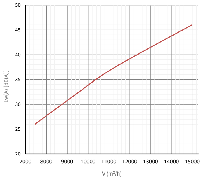
Hangteljesítményszint
