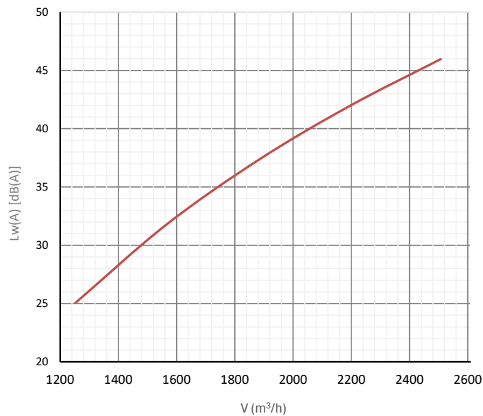
Hangteljesítményszint
