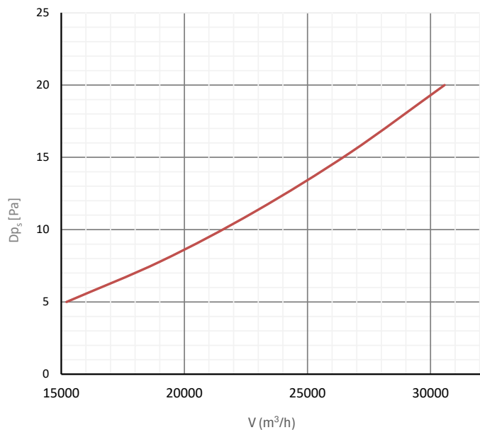
Statikus nyomásveszteség
