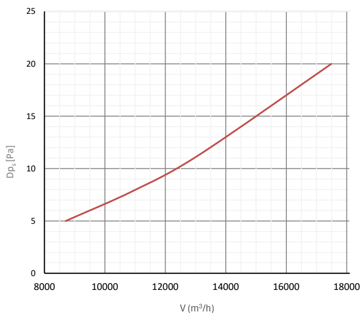
Statikus nyomásvesztés
