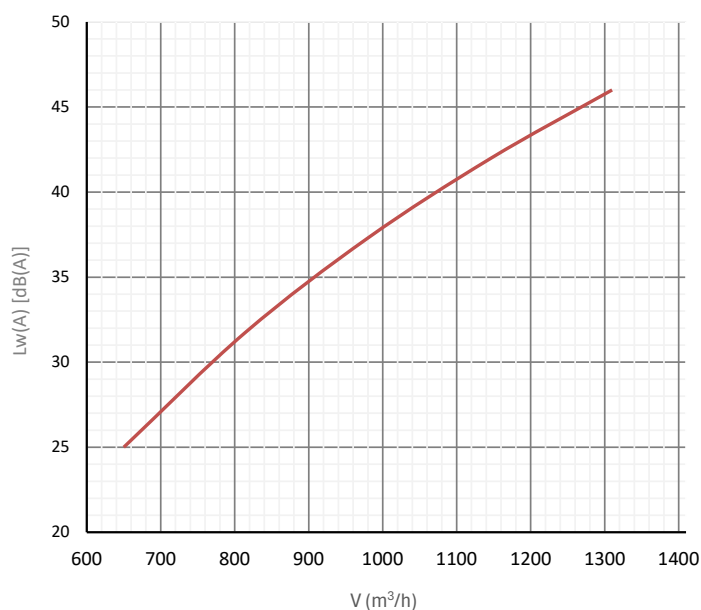
Hangteljesítményszint
