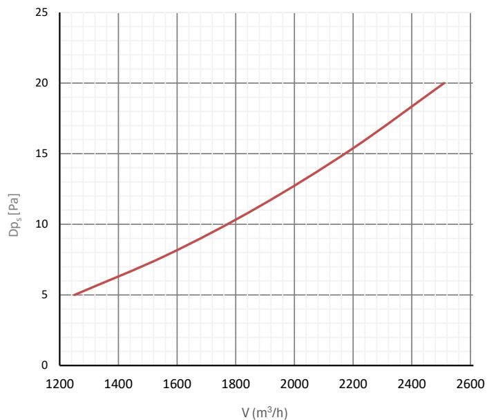
Statikus nyomásveszteség
