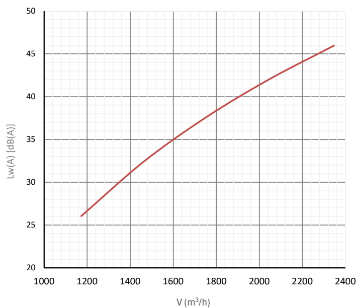
Hangteljesítményszint
