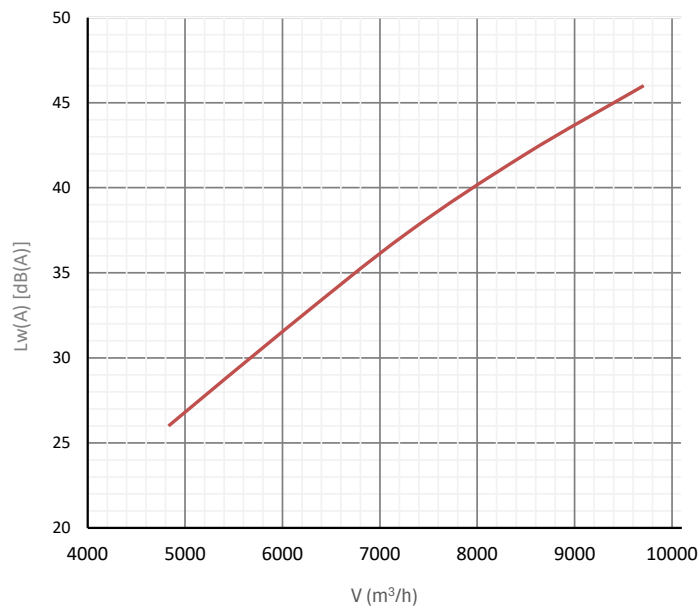
Hangteljesítményszint
