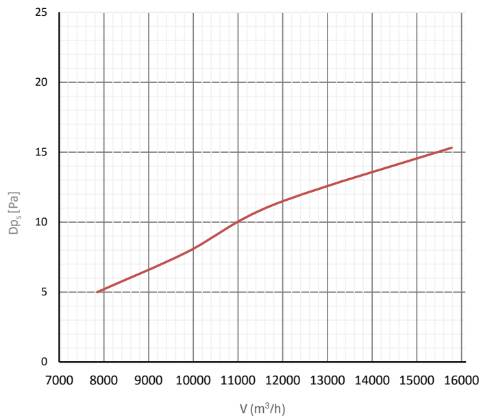
Statikus nyomásvesztés
