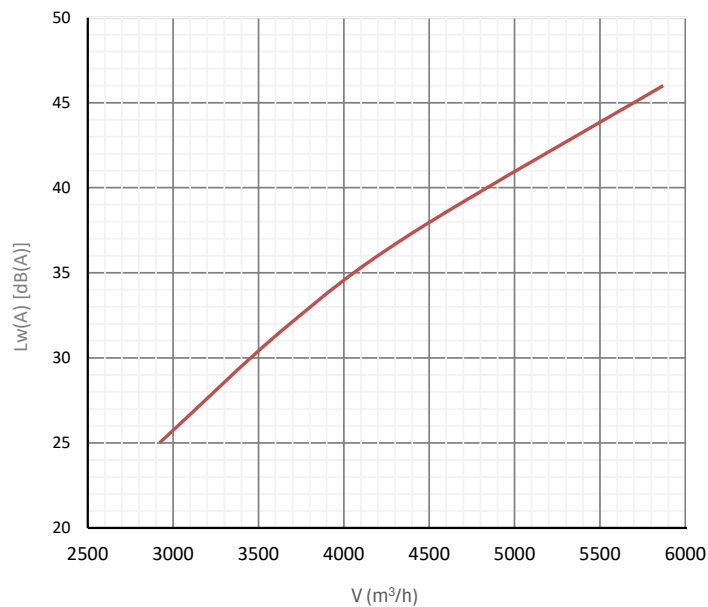
Hangteljesítményszint
