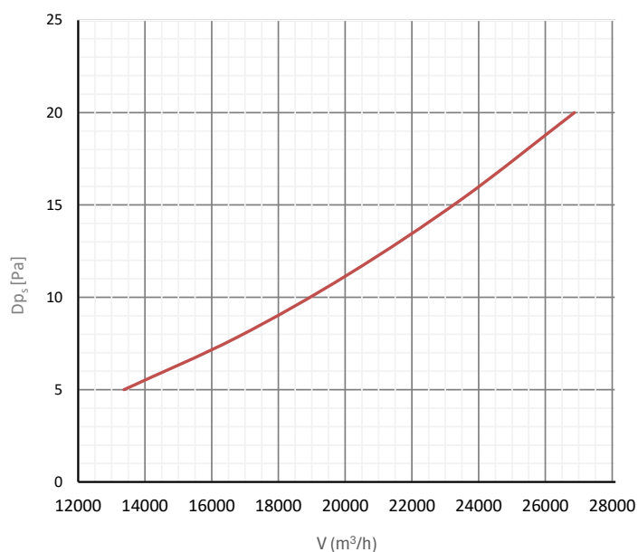
Statikus nyomásveszteség
