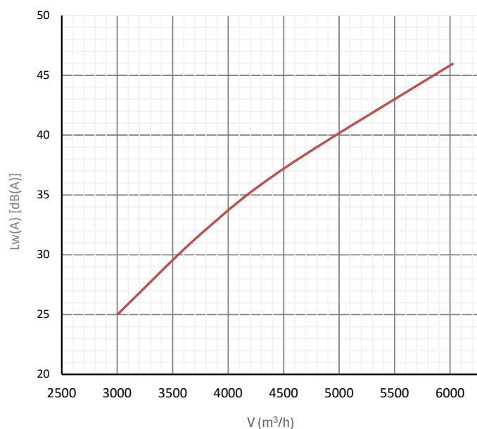
Hangteljesítményszint
