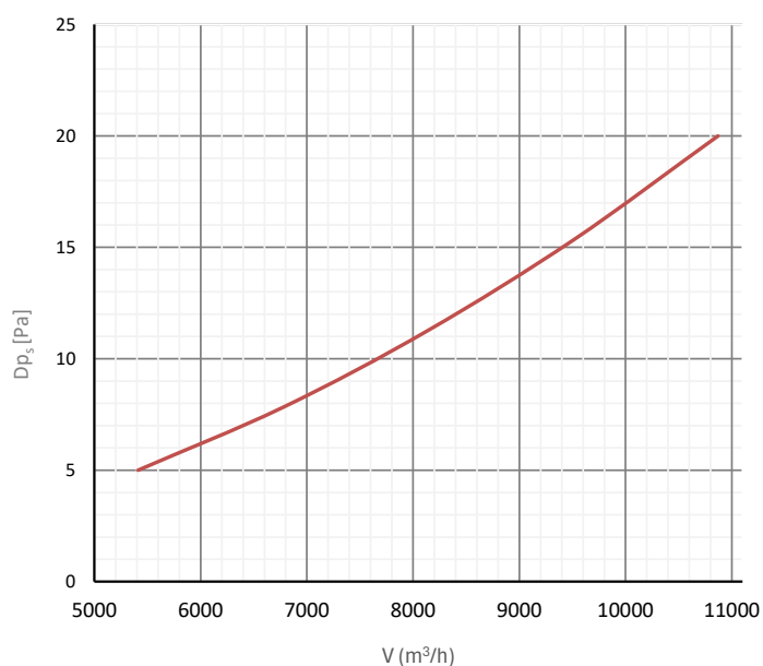
Statikus nyomásvesztés
