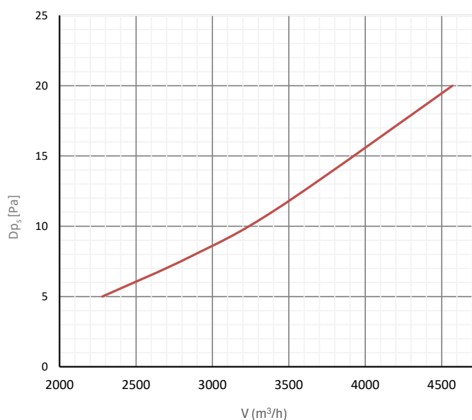
Statikus nyomásvesztés
