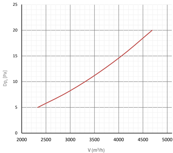
Statikus nyomásveszteség
