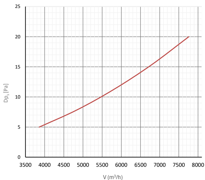
Statikus nyomásvesztés
