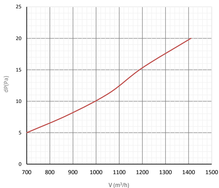
Statikus nyomásvesztés
