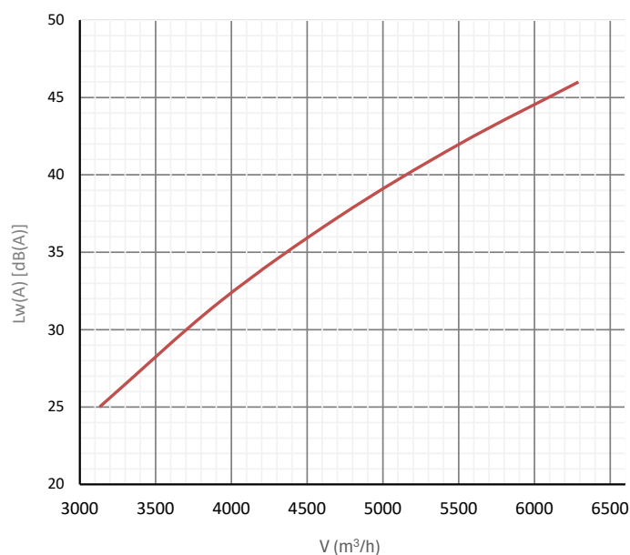
Hangteljesítményszint
