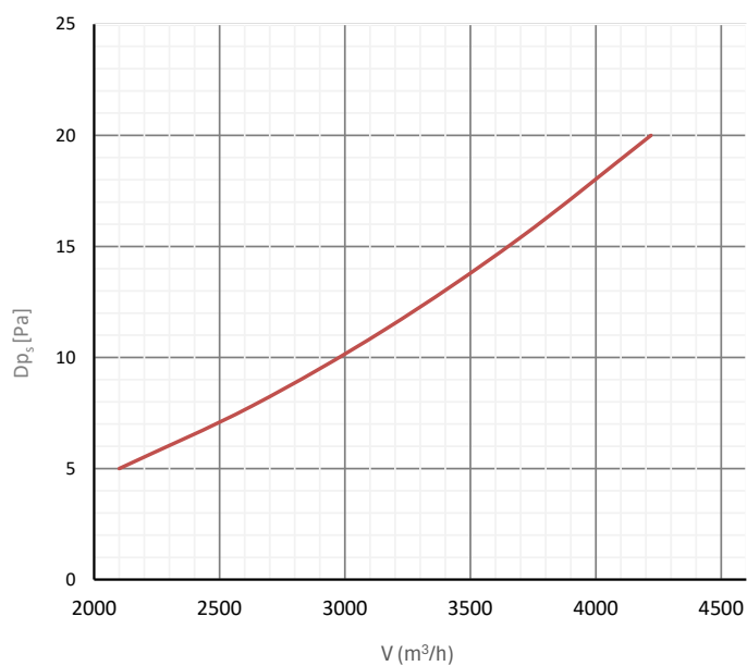
Statikus nyomásvesztés
