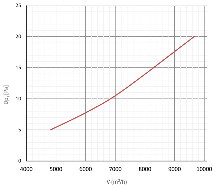
Statikus nyomásvesztés
