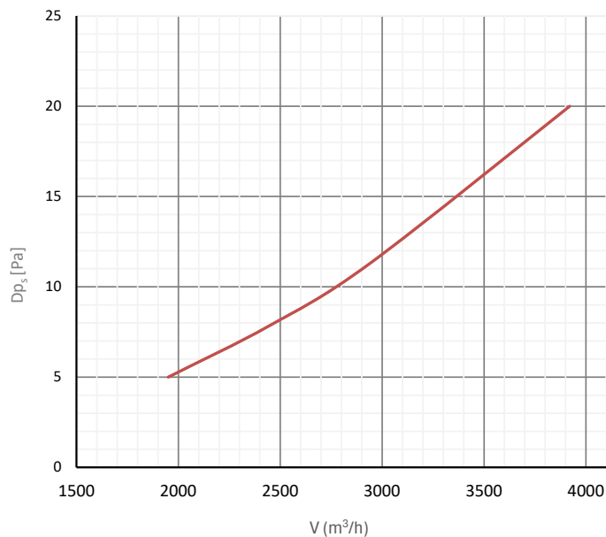
Statikus nyomásvesztés
