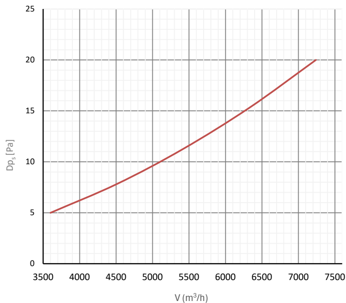
Statikus nyomásvesztés
