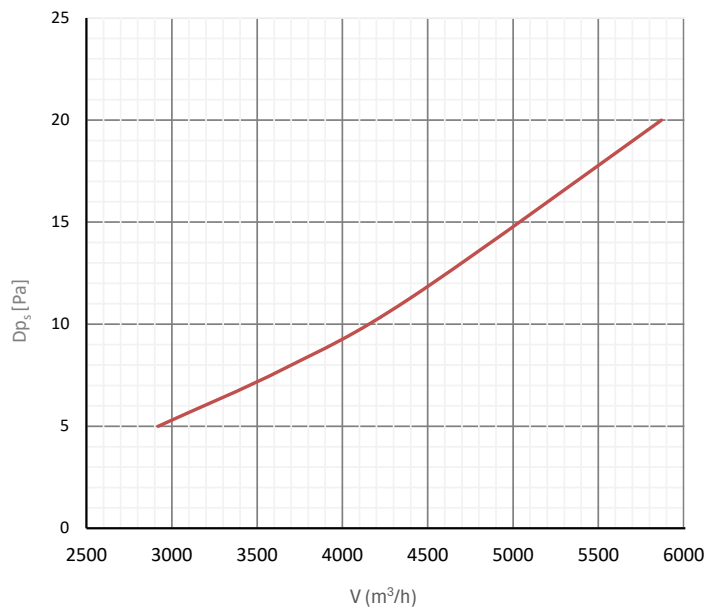
Statikus nyomásveszteség
