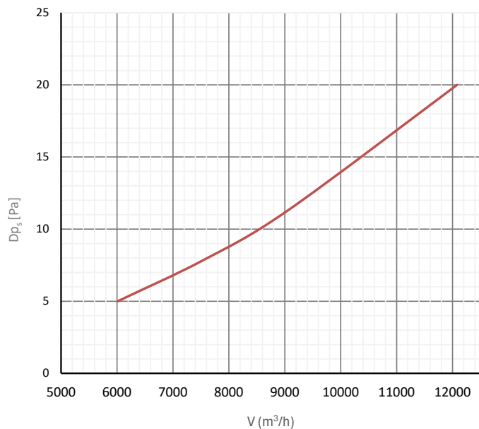
Statikus nyomásvesztés
