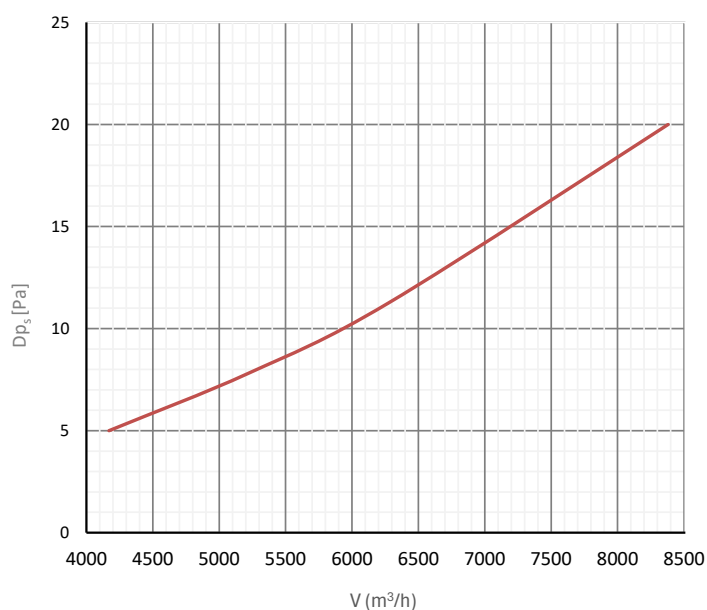
Statikus nyomásveszteség
