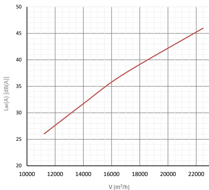
Hangteljesítményszint
