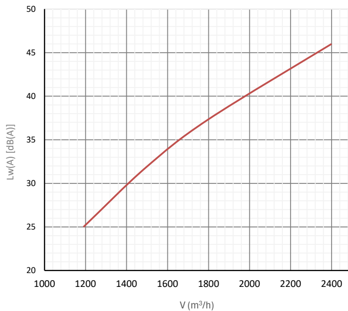
Hangteljesítményszint
