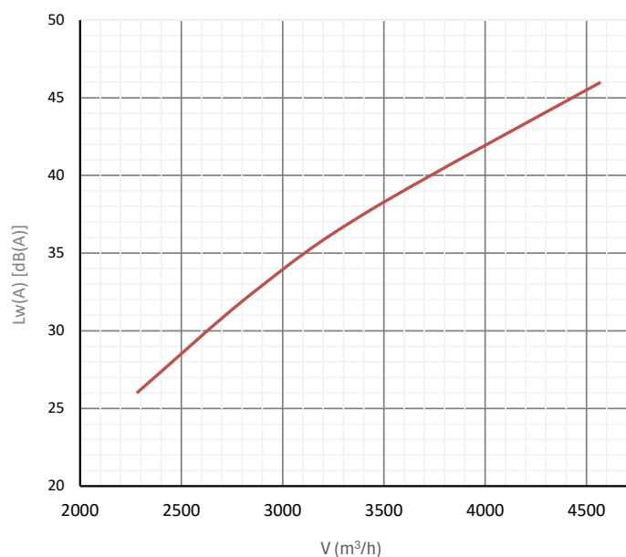
Hangteljesítményszint
