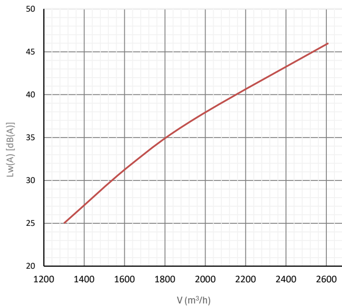
Hangteljesítményszint
