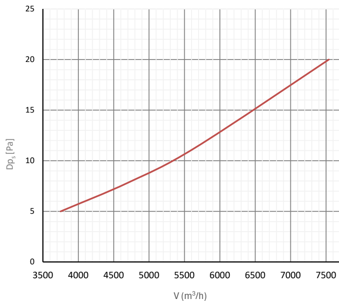
Statikus nyomásveszteség
