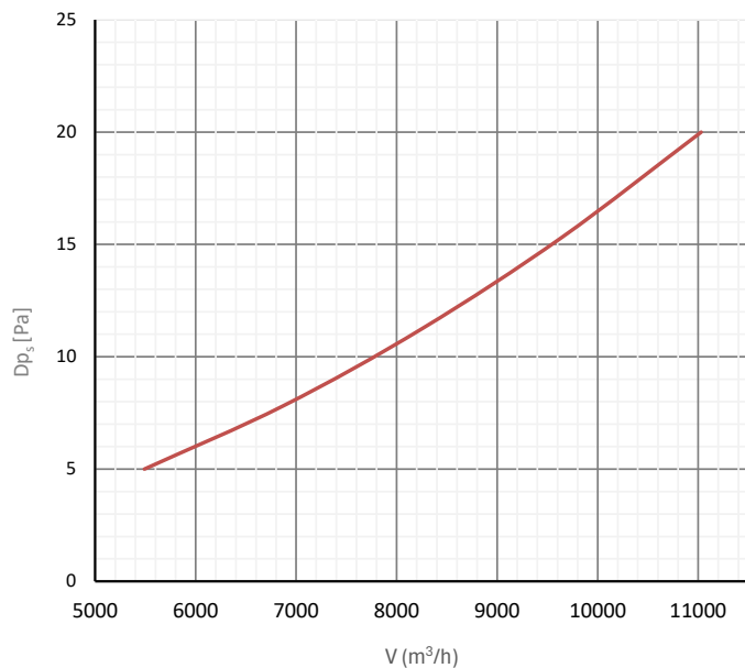
Statikus nyomásvesztés
