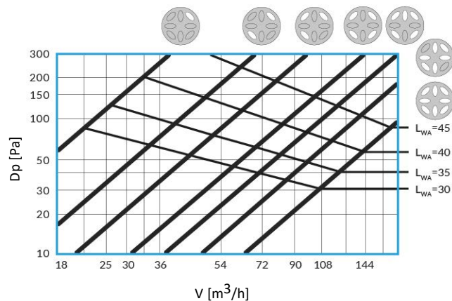
SAVD 125
