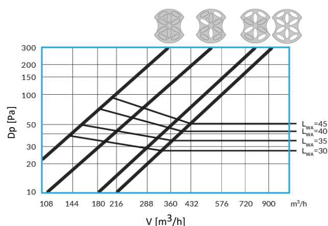
SAVD 315
