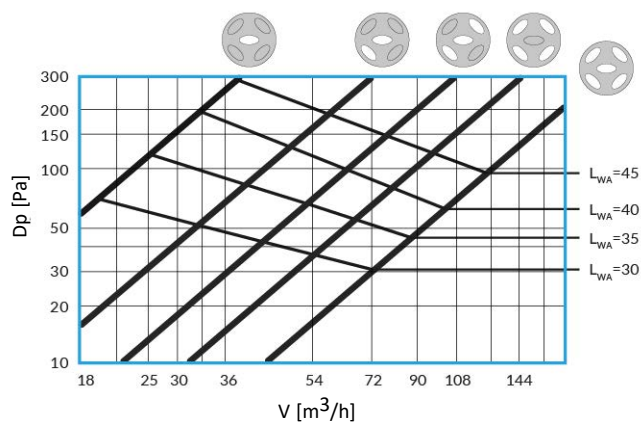
SAVD 100
