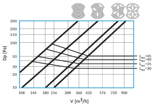
SAVD 250
