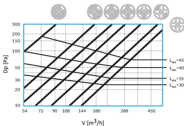
SAVD 200
