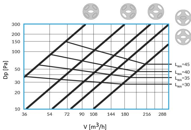
SAVD 160
