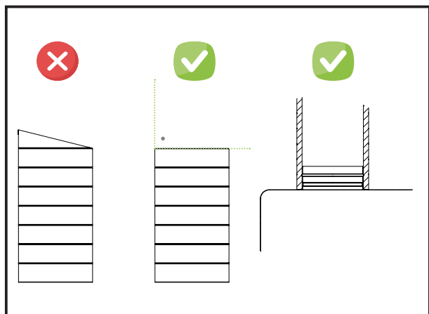
Csatlakozási felület
