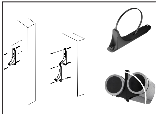
Párhuzamos elhelyezés
