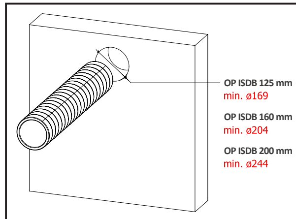
Javasolt falnyílás
