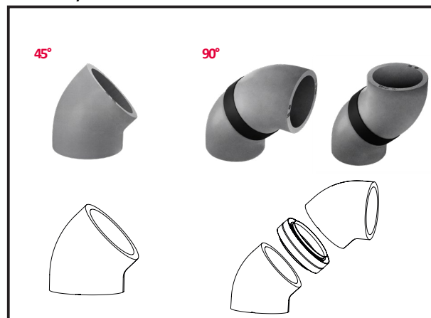
90°-os könyök kialakítása
