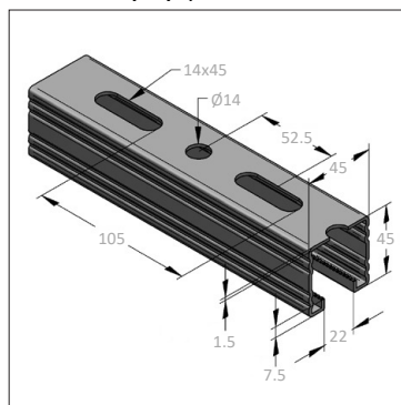
45/45/1,5 szerelőcsín
