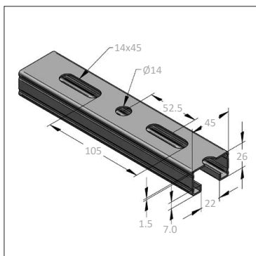
45/26/1,5 szerelőcsín
