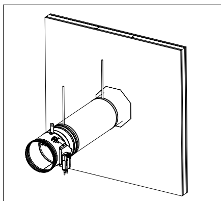
Szerelje fel a tűzvédelmi csappantyút és rögzítse 4,3x10 önmetsző csavarokkal a csatornához (300 mm-enként)
