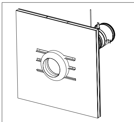
Ismételje meg ugyanezt az eljárást a másik oldalon. Helyezze a gyapjúút a szellőző légcsatornára 80 mm hosszúságban
