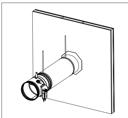
Töltse ki a csatorna és a fal közötti teret ásványgyapattal (Isover U protect, min. 80 mm vastagságú). Ezen kívül a gyapotot 1 mm vastagságban Isover BSF-fel le kell festeni
