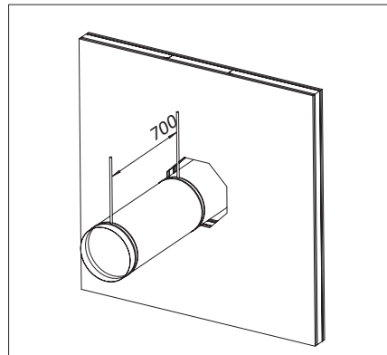
Helyezze a szellőző légcsonnát a falon keresztül (a felfüggesztéshez használt menetes rúd vastagsága legalább M12-s legyen).
