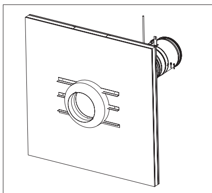
Ismételje meg ugyanezt az eljárást a másik oldalon. Helyezze a gyapút a szellőző légcsonnára 80 mm hosszúságban
