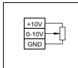
Potenciométer
