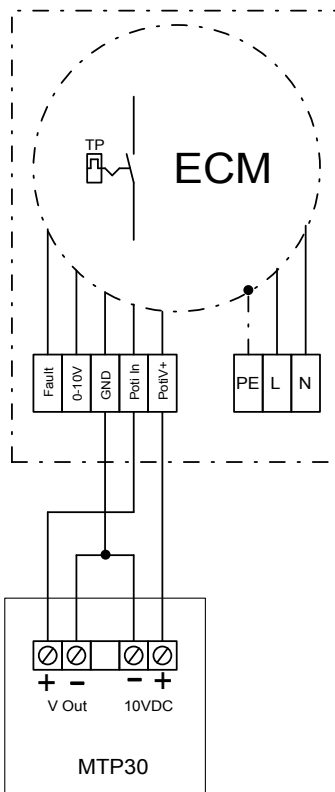
Potenciométer csatlakoztatása MTP30
