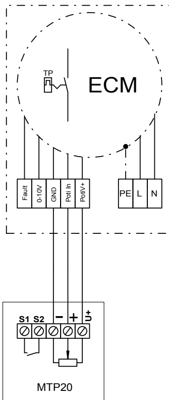
Potenciométer csatlakoztatása MTP20
