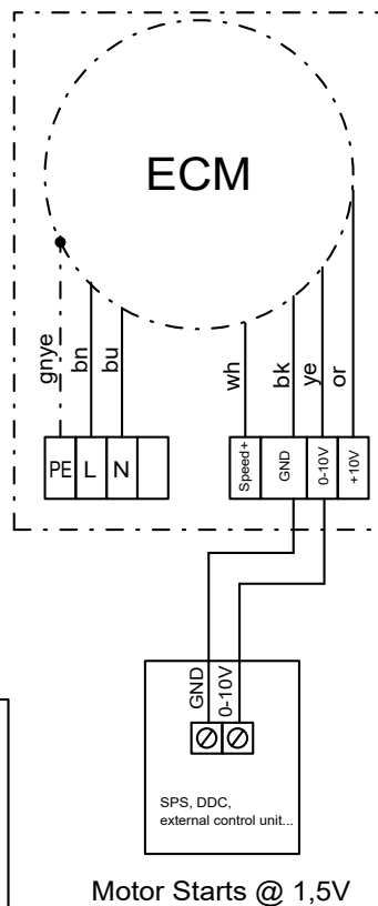
Csatlakoztatás, 0-10 V-os jel
