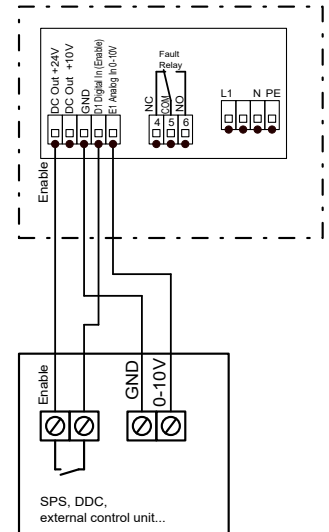
Csatlakoztatás, 0-10 V-os jel
