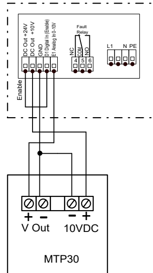
Potenciométer csatlakoztatása MTP30
