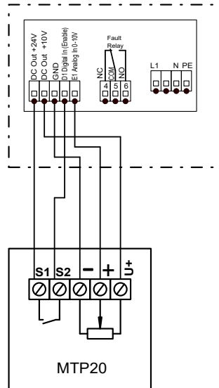
Potenciométer csatlakoztatása MTP20
