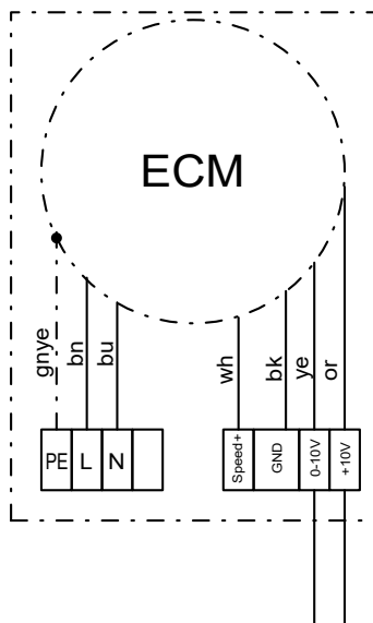
Fordulatszám-szabályozás hiánya 100%-os teljesítmény
