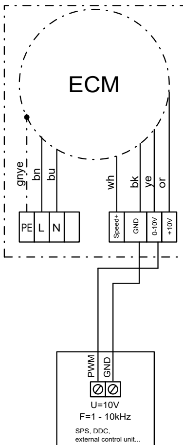
Csatlakozás PWM jellel
