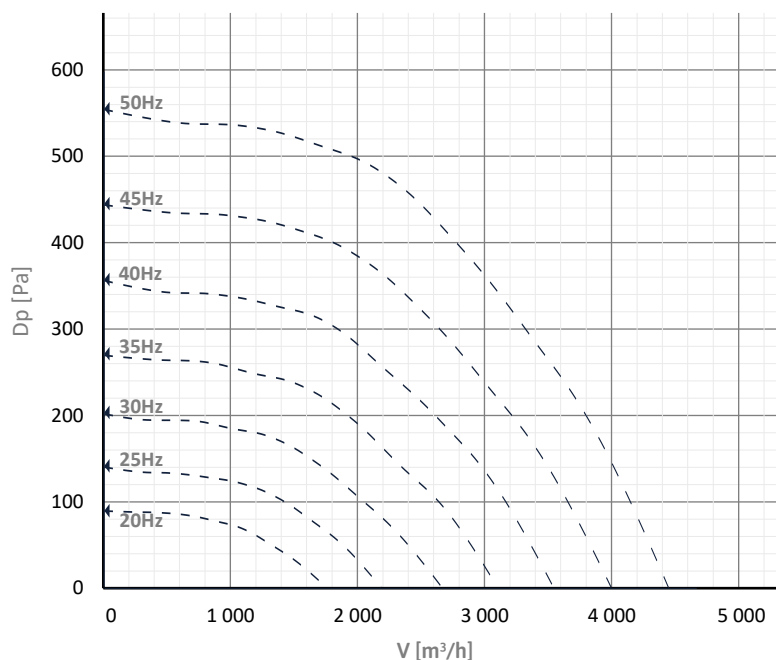
KCF-N 400 D4 40
