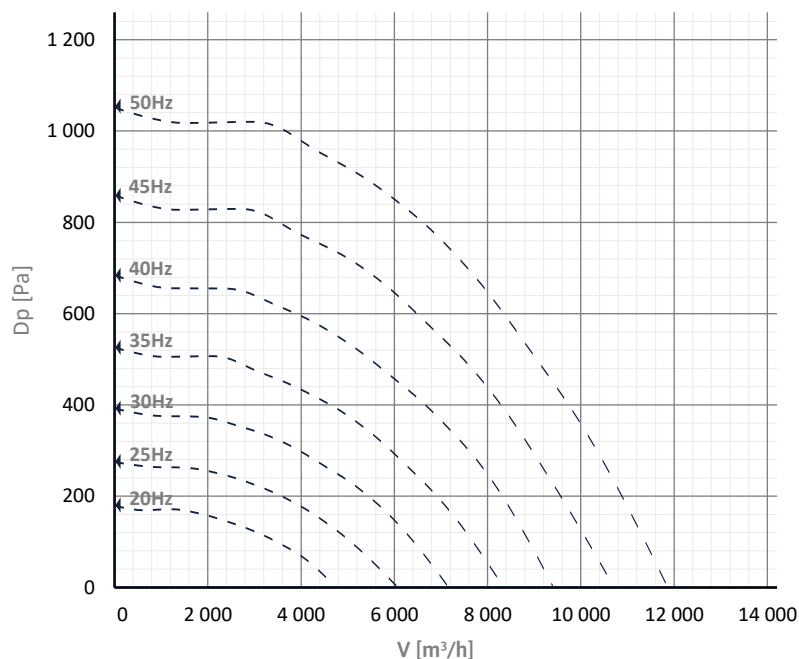
KCF-N 560 D4 40
