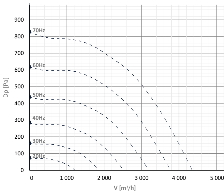
KCF-N 355 D4 40
