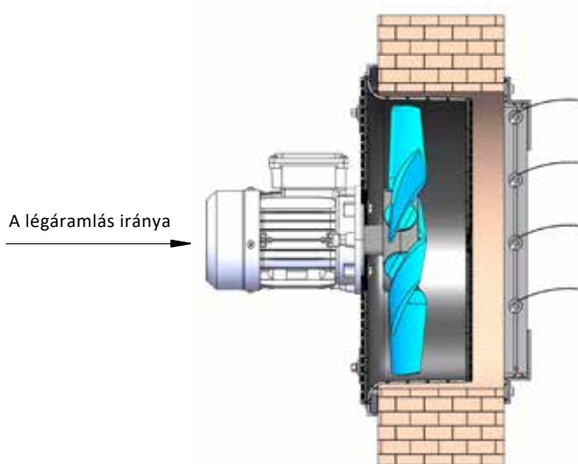
FALBA TÖRTÉNŐ ELHELYEZÉS
