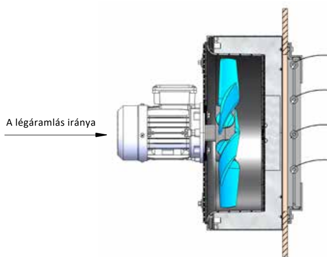
FALSÍKRA VALÓ ELHELYEZÉS TÁVOLSÁGTARTÓVAL
