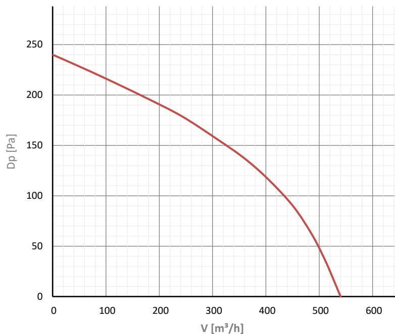
CFV 160
