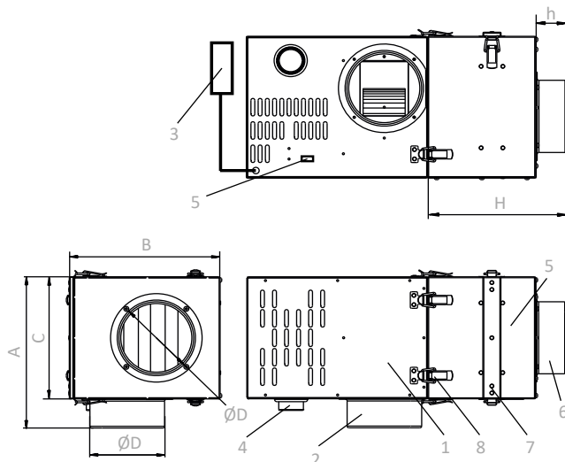
Kandalló ventilátor CFV-FF szűrőelemmel
