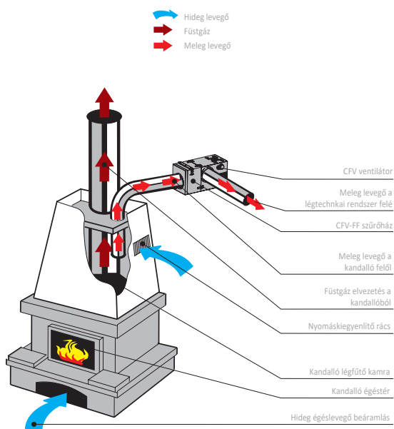
CFV-FF szűrőmodullal felszerelt CFV ventilátor beépítése a kéményrendszerbe
