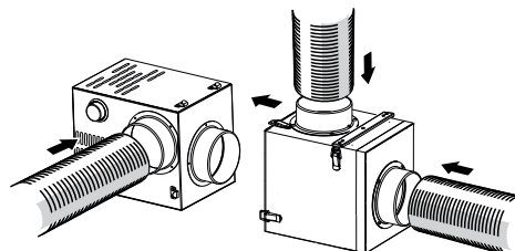
CFV-FF szűrőmodul és flexibilis cső csatlakoztatása
