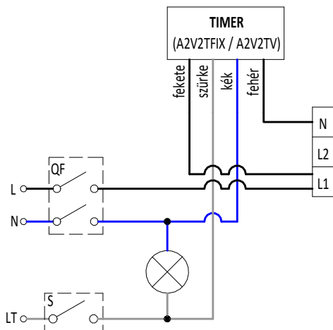
2 fokozatú ventilátor bekötés (minimum fokozat)
