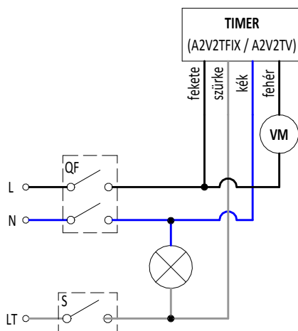
Általános bekötés
