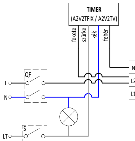
2 fokozatú ventilátor bekötés (maximum fokozat)
