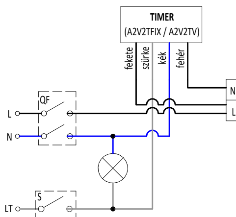
1 fokozatú ventilátor bekötés
