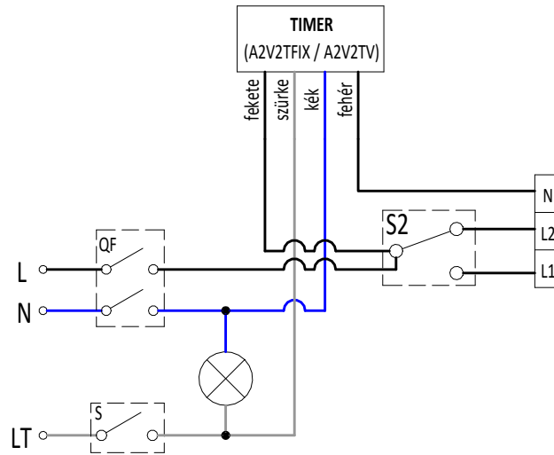
2 fokozatú ventilátor bekötés (fokozatkapcsolóval)
