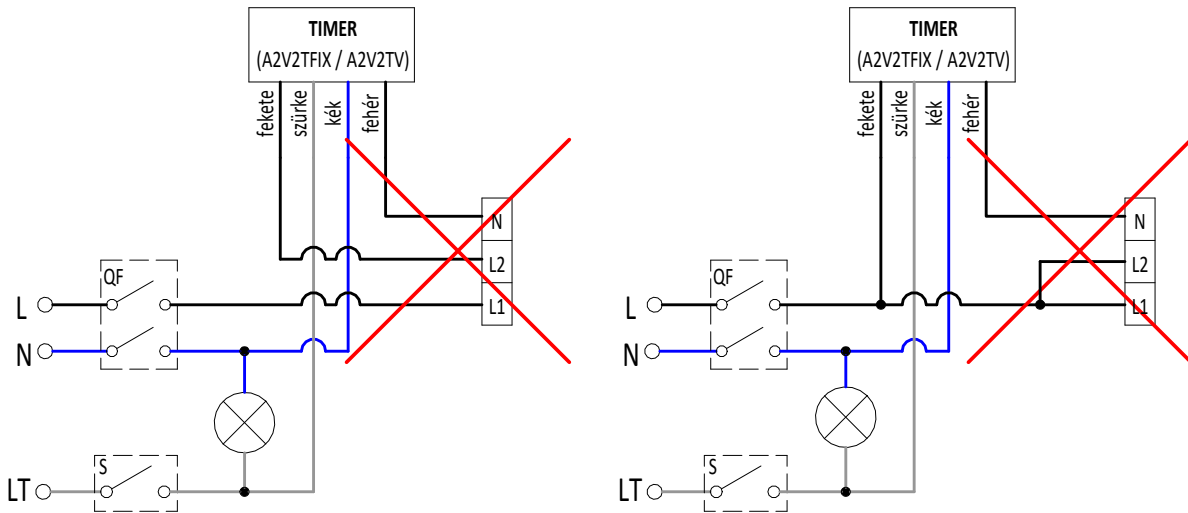
2 fokozatú ventilátor hibás bekötések
