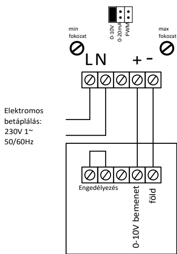
Frekvenciszabályzó 0-10V bemenet
