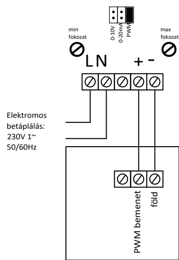
EC-Motor PWM bemenet
