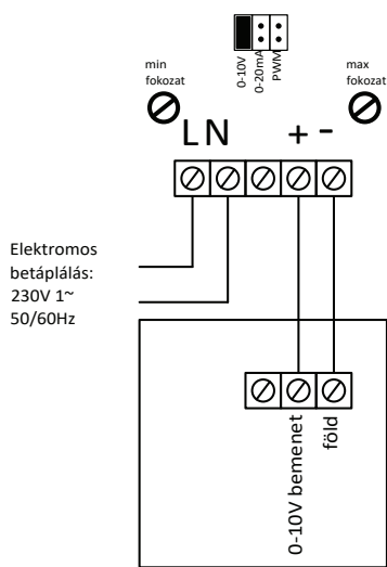
EC-Motor 0-10V bemenet
