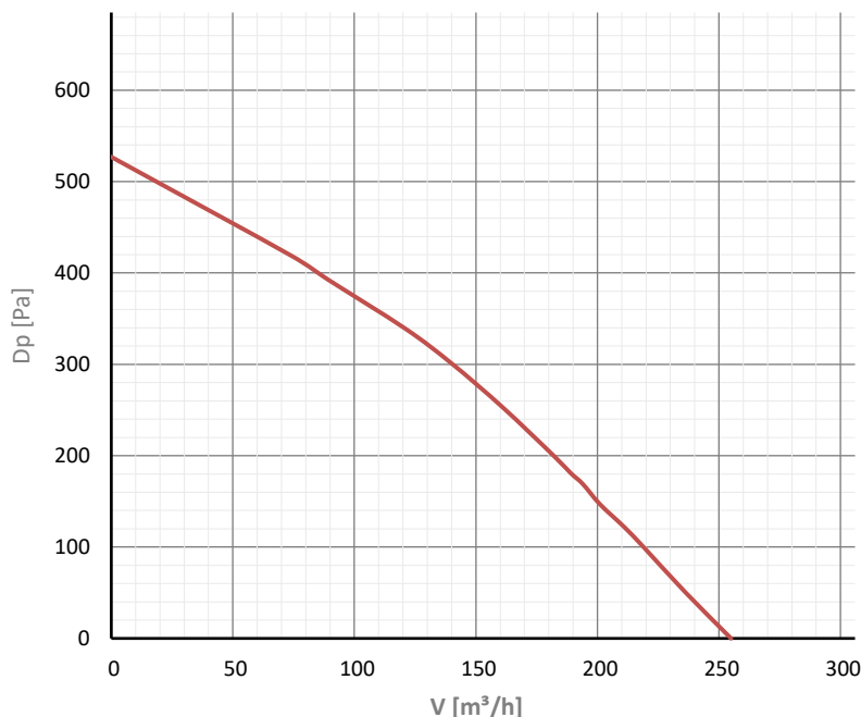
HRS Smarty 2X C 1.1 Befúvás max
