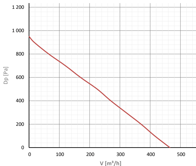
HRS Smarty 3X C 1.1 Elszívás max
