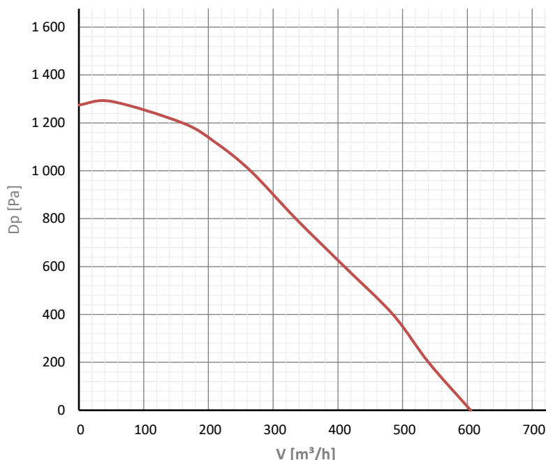
HRS Smarty 4X C 1.1 Befúvás max
