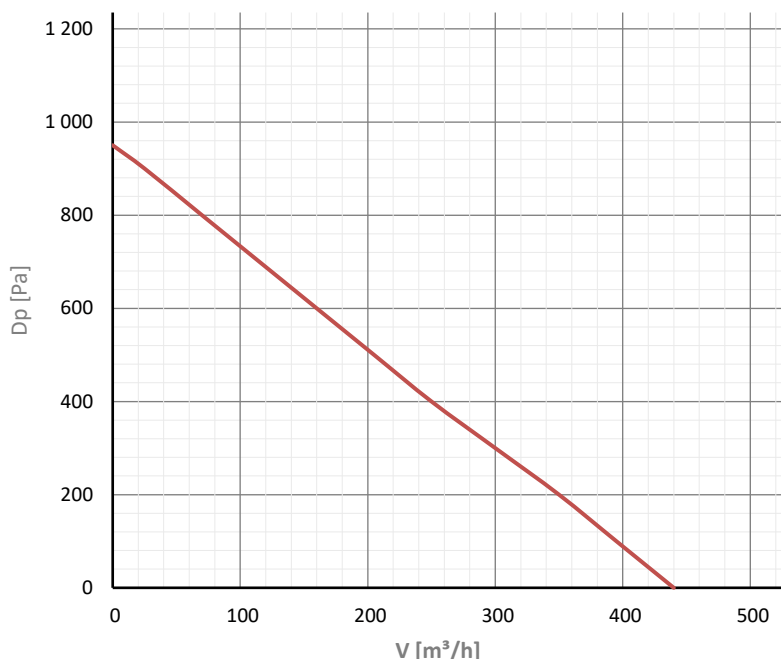
HRS Smarty 3X C 1.1 Befúvás max
