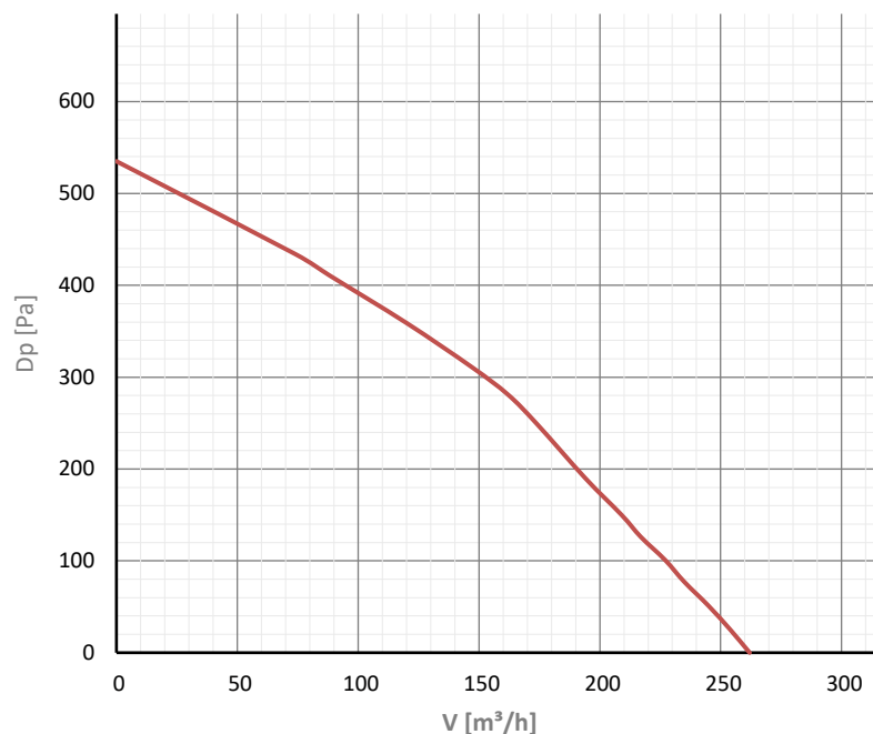
HRS Smarty 2X C 1.1 Elszívás max
