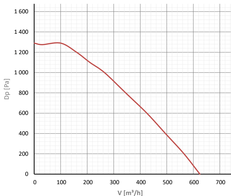
HRS Smarty 4X C 1.1 Elszívás max
