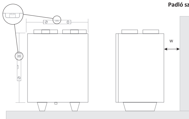
Vízszintes szerelési pozíció a padlón. (W=400mm) padlón
