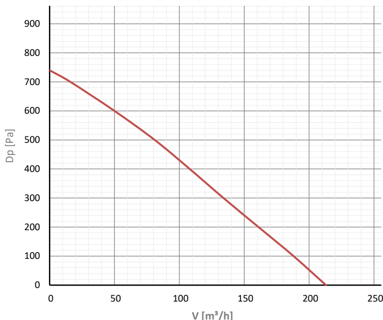
HRS Smarty 2X V 1.1 Befúvás max
