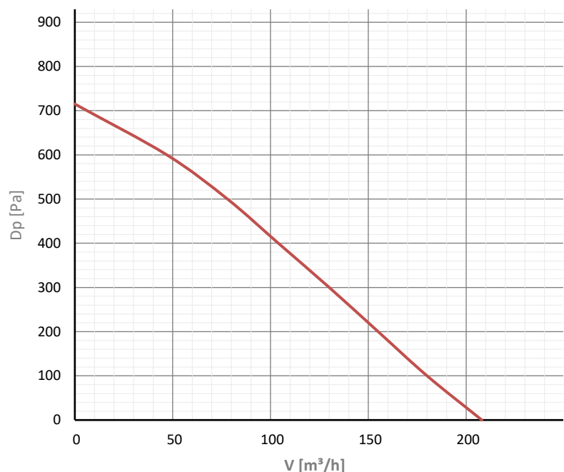
HRS Smarty 2X V 1.1 Elszívás max
