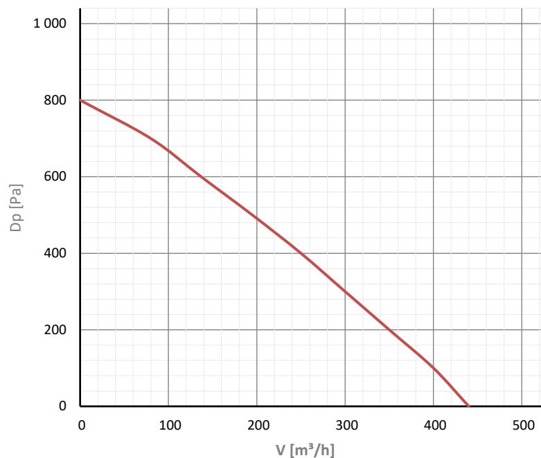
HRS Smarty 3X V 1.1 Elszívás max
