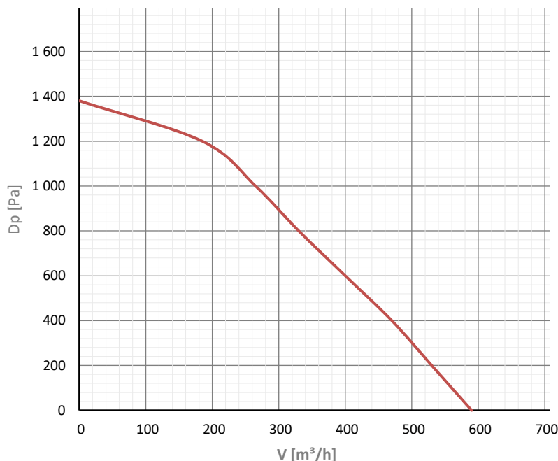
HRS Smarty 4X V 1.1 Befúvás max
