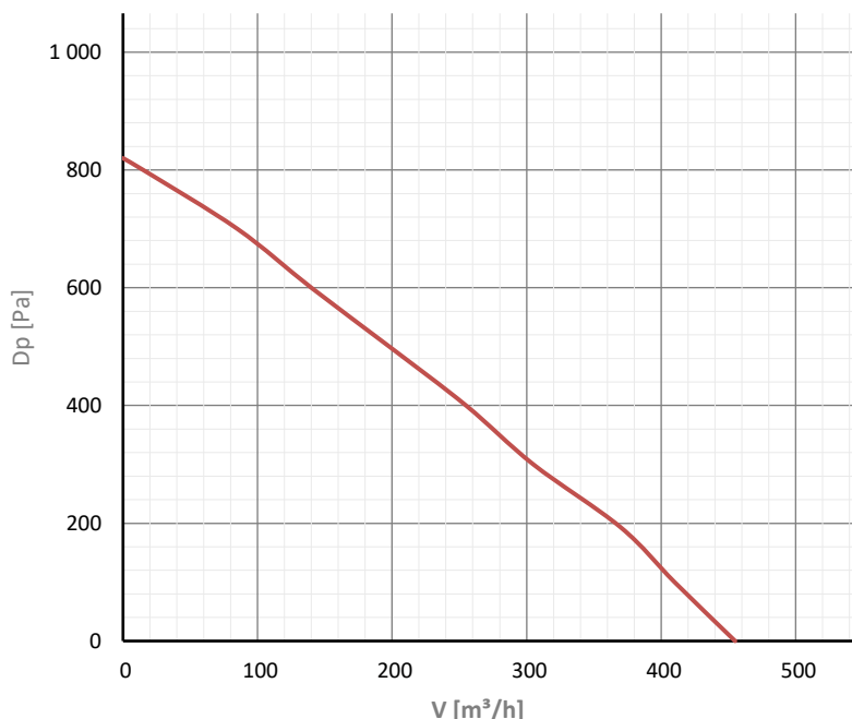
HRS Smarty 3X V 1.1 Befúvás max
