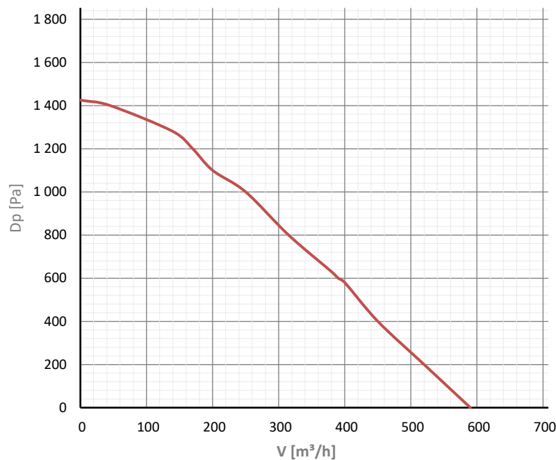
HRS Smarty 4X V 1.1 Elszívás max
