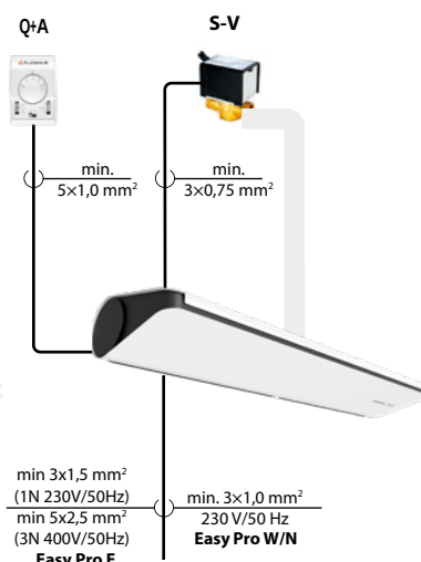
elektromos betáplálás
