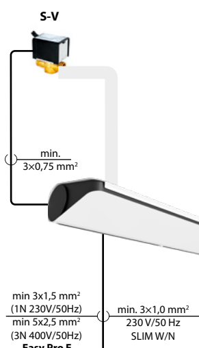
elektromos betáplálás
