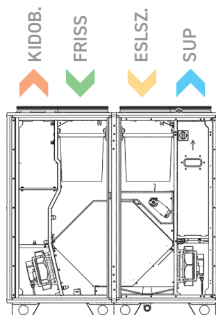
AmberAir Compact S-CXV (jobbos)
