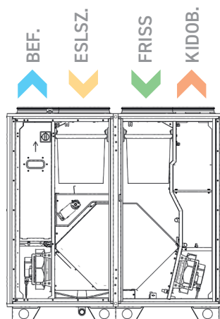
AmberAir Compact S-CXV (balos)
