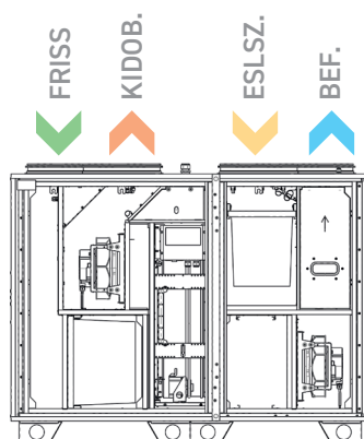
AmberAir Compact S-RV (jobbos)
