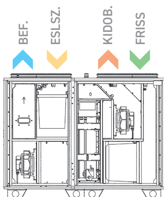
AmberAir Compact S-RV (balos)
