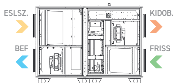
AmberAir Compact S-RH (balos)
